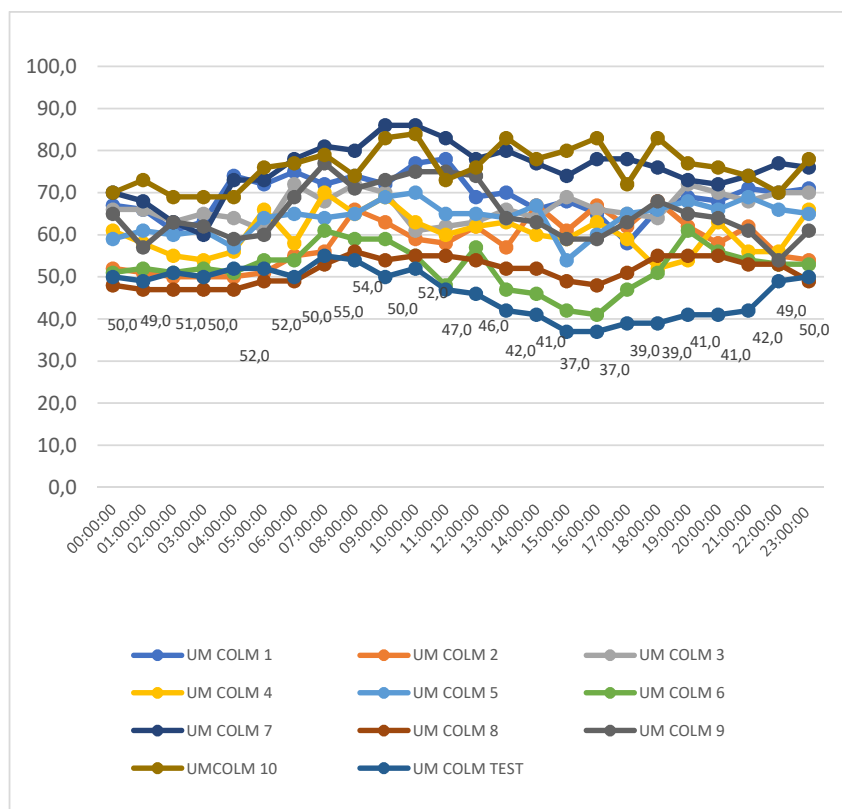
Gráfico 17 - Umidades e suas oscilações registradas nas colmeias povoadas e na colmeia testemunha, nas 24 (vinte e quatro) horas do dia 22 de outubro de 2021 Fonte: Autor (2022)
