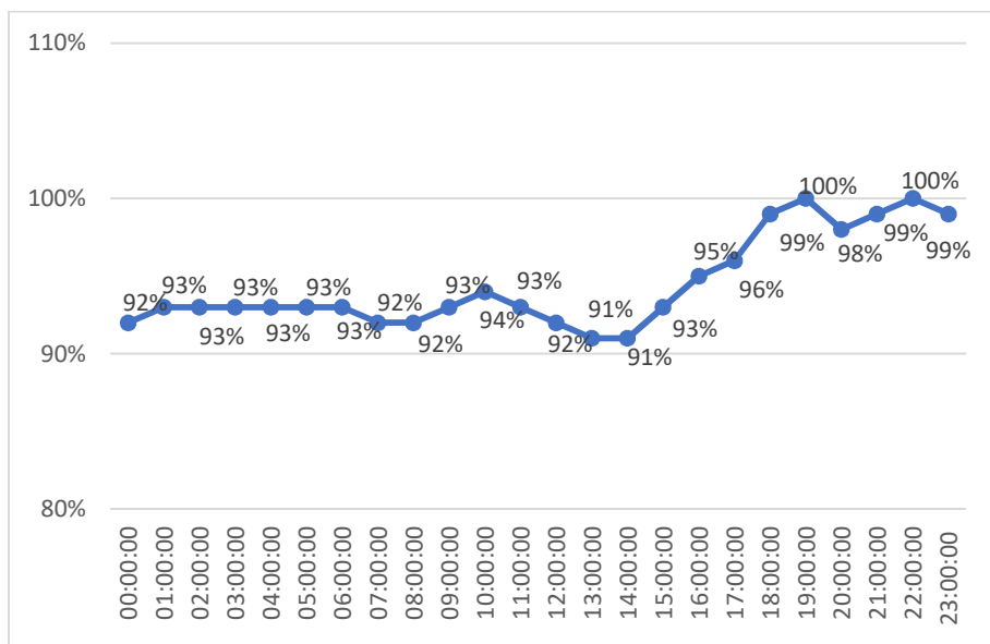
Gráfico 36 - Variação da umidade na colmeia 11 (testemunha) em 20/03/2022
