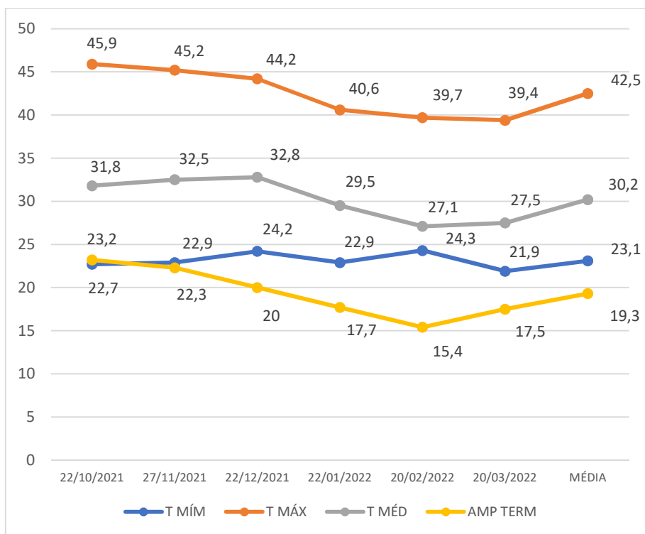
Gráfico 10 - Temperaturas mínima, máxima e média registradas no ambiente do apiário, de outubro de 2021 a março de 2022 e a média do semestre
