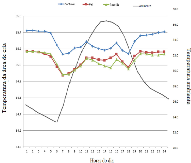
Gráfico 2 – Média das temperaturas do ambiente externo e das colônias Apis mellifera (hymenoptera: apidae) em todos os tratamentos num período de 24 horas, 2016
