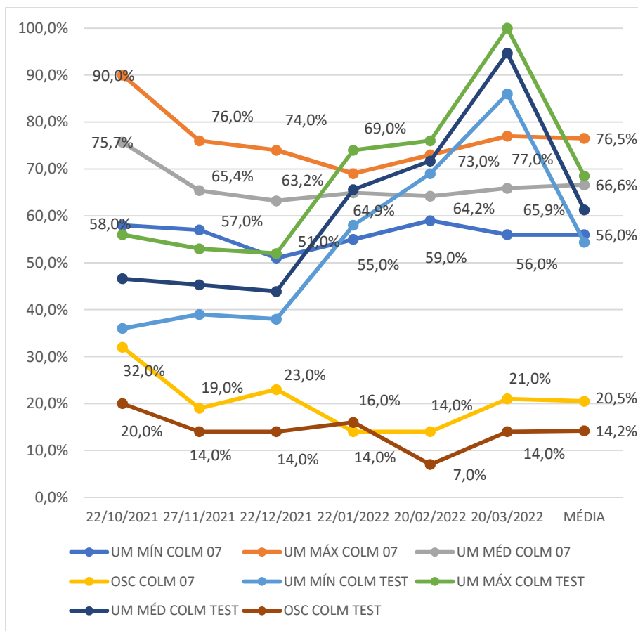
Gráfico 51 - Umidades registradas na colmeia 7 (povoada) e na colmeia 11 (testemunha), de out/2021 a mar/2022
