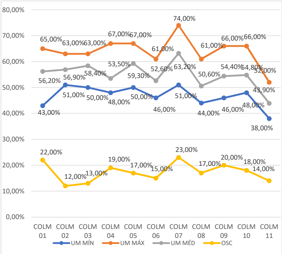
Gráfico 66 - Umidades mínima, máxima, média e as respectivas oscilações da umidade na colmeia testemunha, e nas dez colmeias povoadas, em 22/12/2022 Fonte: Autor (2022)
