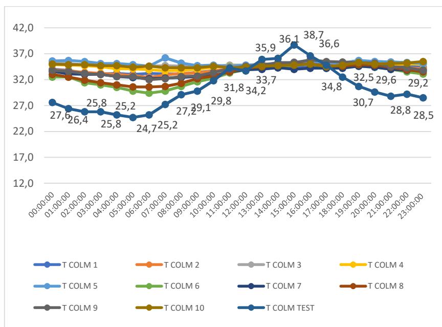
Gráfico 15 - Temperaturas e suas oscilações registradas nas colmeias povoadas e na colmeia testemunha, nas 24 (vinte e quatro) horas do dia 22 de outubro de 2021
