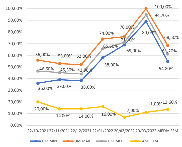
Gráfico 7 - Umidades mínima, máxima e média registradas na colmeia 11, de outubro de 2021 a março de 2022 (três meses secos e três meses chuvosos) e a média do semestre Fonte: Autor (2022)
