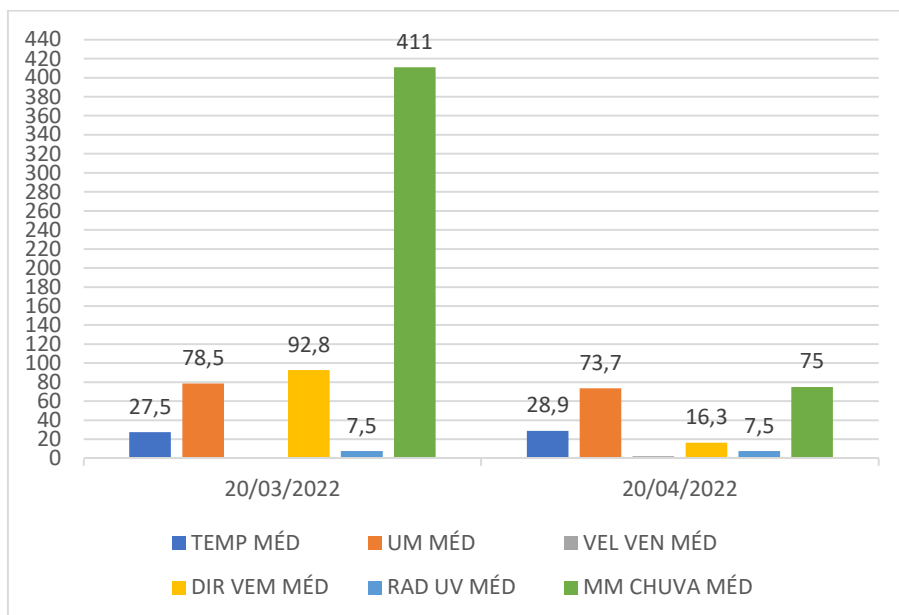
Gráfico 5 - Médias de temperatura, umidade, direção do vento, velocidade do vento, radiação UV e mm de chuva registradas pelas estações 01 e 02 em 20/03/2022 e 20/04/2022 no ambiente do apiário
