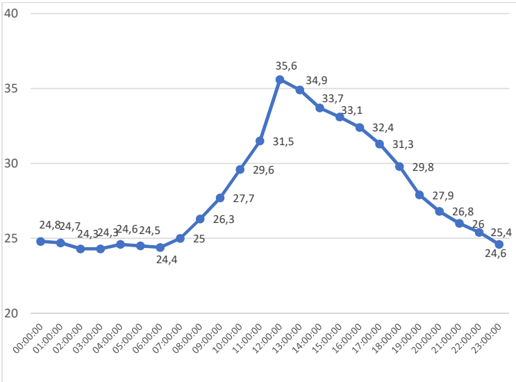
Gráfico 26 - Variação da temperatura na colmeia 11 (testemunha) em 22/01/2022 Fonte: Autor (2022)
