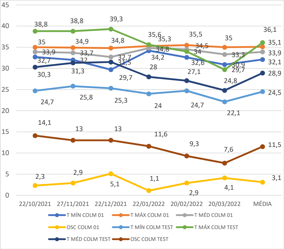
Gráfico 38 - Temperaturas registradas nas colmeias 1 e na colmeia 11 (testemunha) de out/2021 a mar/2022 Fonte: Autor (2022)
