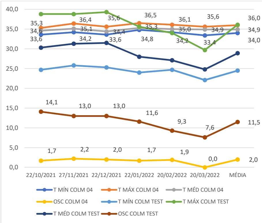
Gráfico 44 - Temperaturas registradas na colmeia 4 (povoada) e na colmeia 11 (testemunha) de out/2021 a mar/2022 Fonte: Autor (2022)
