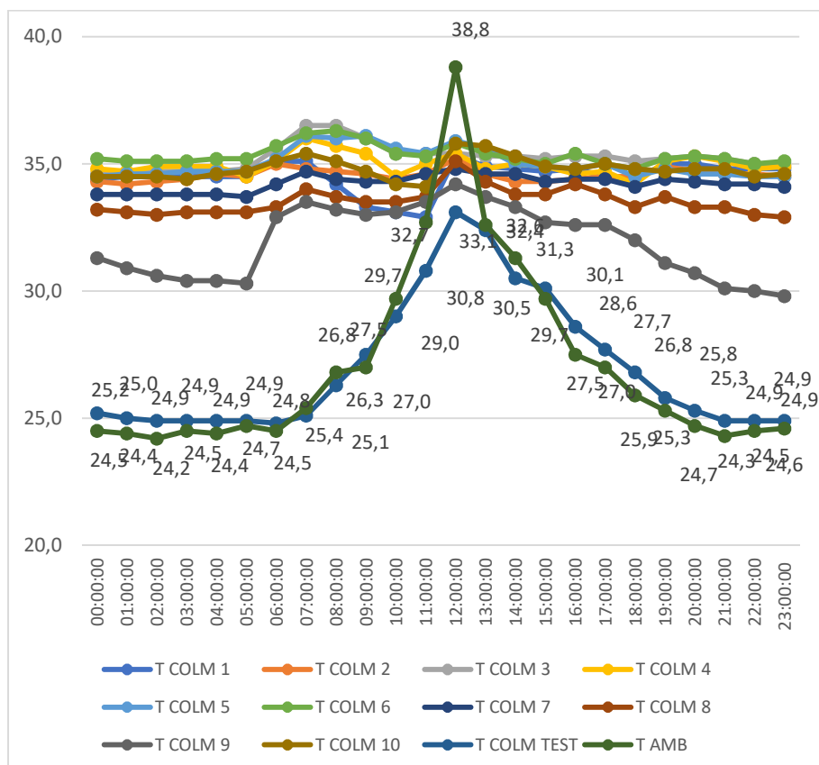
Gráfico 31 - Temperaturas e suas oscilações registradas nas colmeias povoadas, na colmeia testemunha e no ambiente, nas 24 (vinte e quatro) horas do dia 20 de fevereiro de 2022
