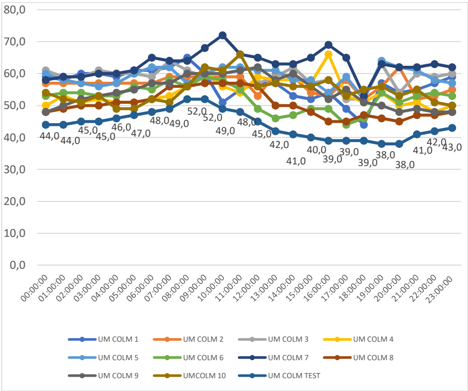
Gráfico 25 - Umidades e suas oscilações registradas nas colmeias povoadas e na colmeia testemunha, nas 24 (vinte e quatro) horas do dia 22 de dezembro de 2021 Fonte: Autor (2022)
