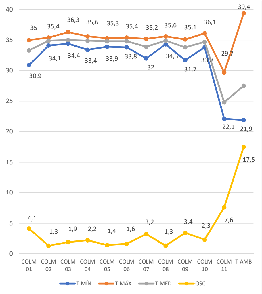
Gráfico 63 - Temperaturas mínima, máxima, média e as respectivas oscilações da temperatura na colmeia testemunha, no ambiente e nas dez colmeias povoadas, em 20/03/2022 Fonte: Autor (2022)
