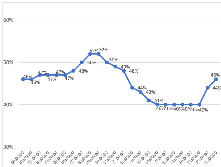
Gráfico 20 - Oscilação da umidade na colmeia 11(testemunha) em 27/11/2021 Fonte: Autor (2022)
