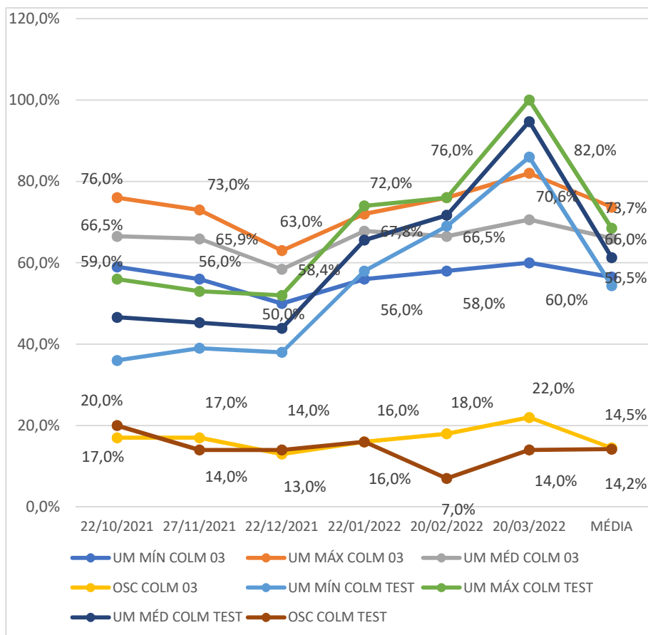
Gráfico 43 - Umidades registradas nas colmeias 3 (povoada) e na colmeia 11 (testemunha) de out/2021 a mar/2022 Fonte: Autor (2022)
