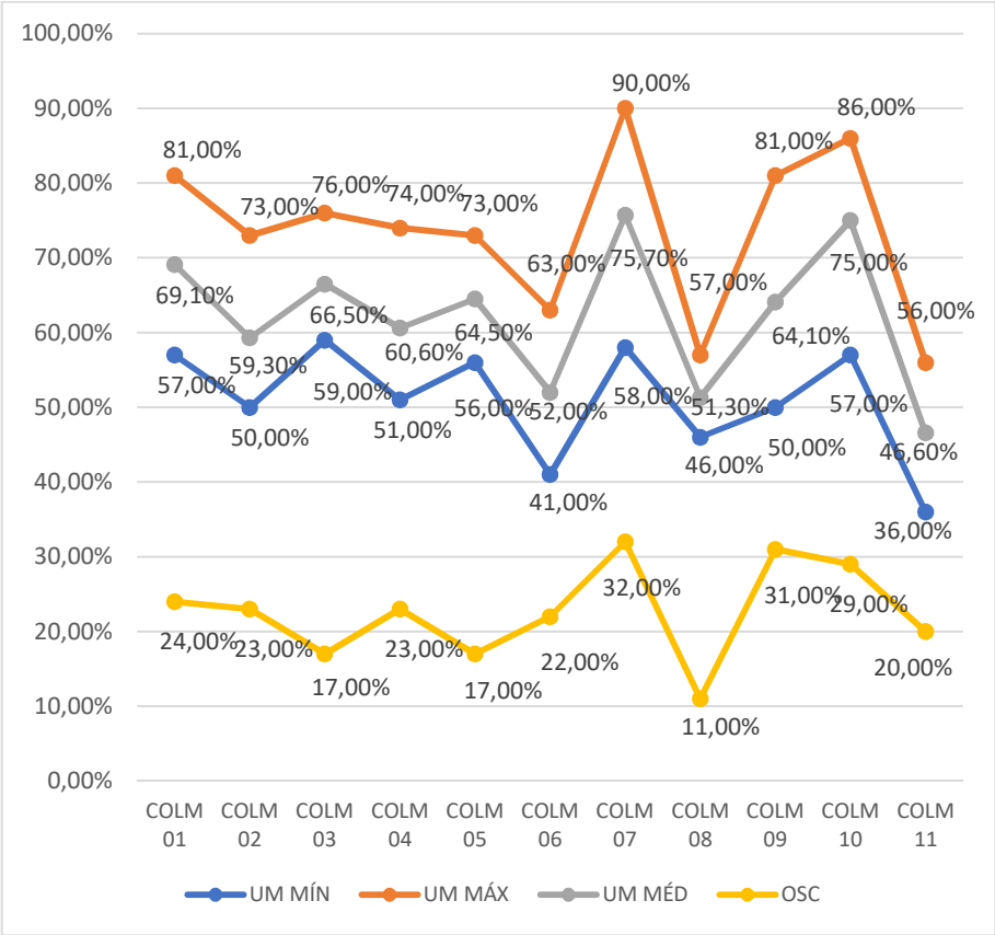
Gráfico 64 - Umidades mínima, máxima, média e as respectivas oscilações da umidade na colmeia testemunha, e nas dez colmeias povoadas, em 22/10/2022 Fonte: Autor (2022)
