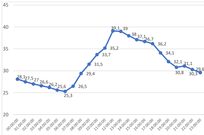
Gráfico 22 - Variação da temperatura na colmeia 11 (testemunha) em 22/12/2021 Fonte: Autor (2022)
