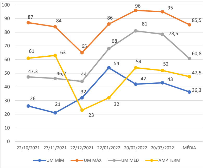
Gráfico 11 - Médias das umidades mínima, máxima, média e oscilação da umidade (%), registradas nos meses de out/21 a mar/22, no ambiente do apiário e a média desse semestre
