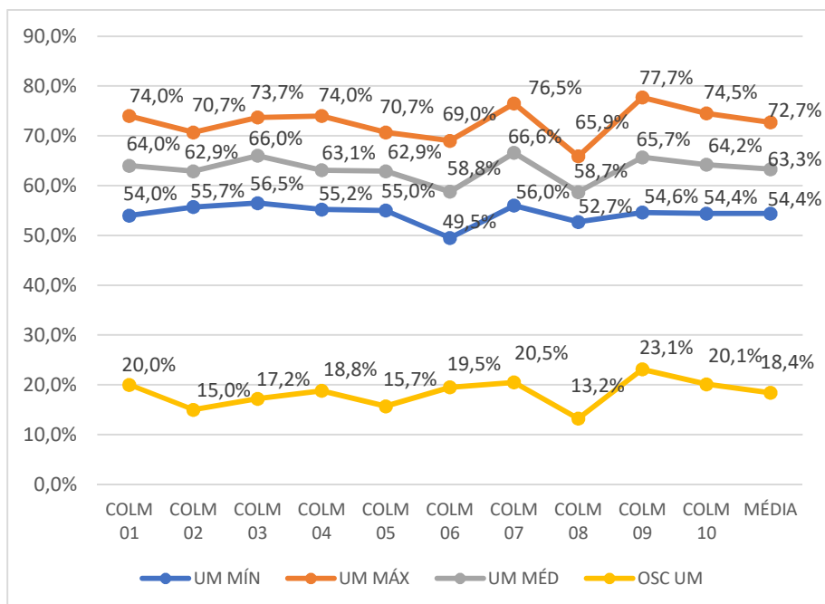
Gráfico 71 - Médias de umidade mínima, máxima, média e a oscilação de umidade, com dados dos seis meses pesquisados, das 10 colmeias para determinação da zona de conforto térmico no ninho da Apis mellifera L.
