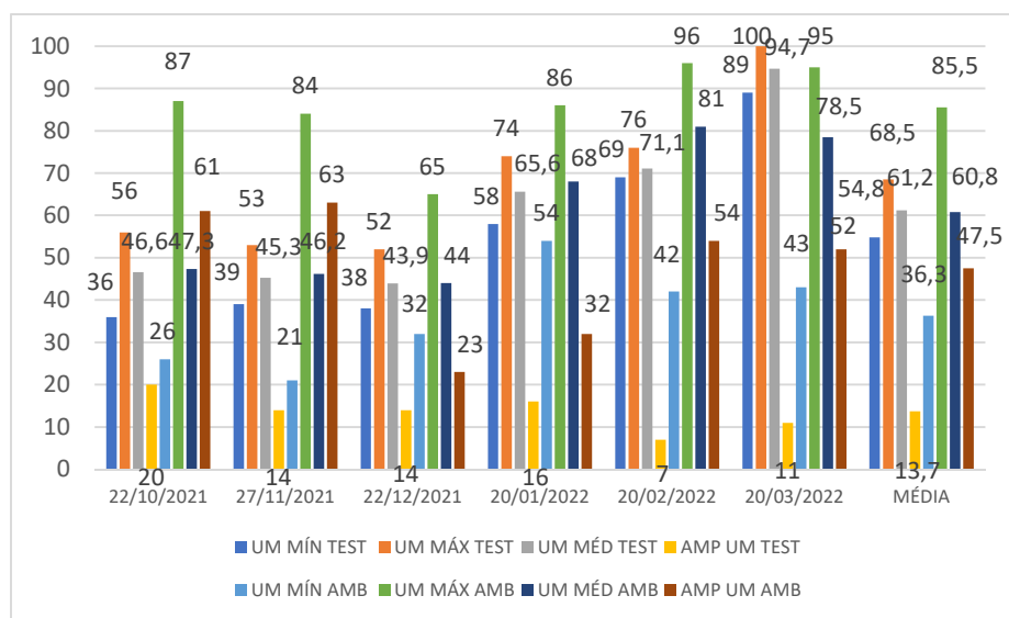
Gráfico 13 - Médias de umidades mínima, máxima, média e oscilação da umidade (%) na colmeia 11 (testemunha) e no ambiente do apiário, no período de out/2021 a mar/2022.
