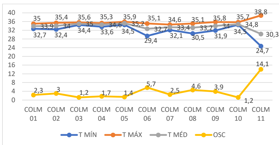
Gráfico 58 - Temperaturas mínima, máxima, média e as respectivas oscilações da temperatura na colmeia testemunha e nas dez colmeias povoadas, em 22/10/2021
