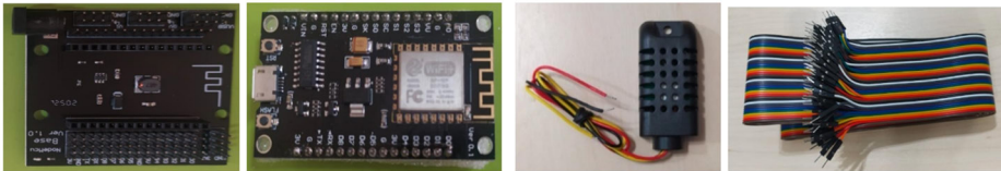
Figura 11 – Shield base de alimentação para esp 8266 nodemcu, módulo Wi-Fi esp8266 nodemcu v3 (ch340), sensor dht 21 de temperatura/umidade e jumper fio dupont conector para ESP 8266 male female 100 cm
