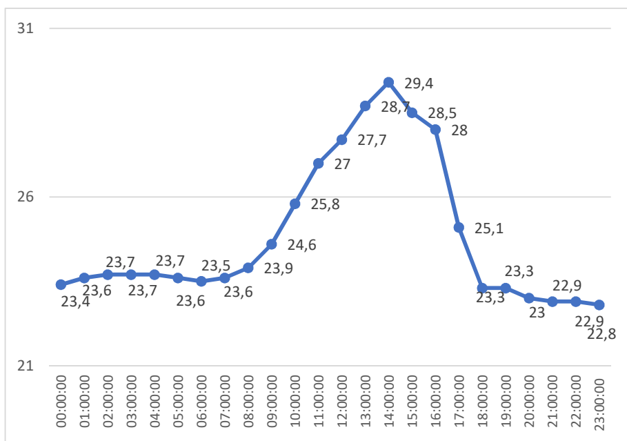
Gráfico 34 - Variação da temperatura na colmeia 11 (testemunha) em 20/03/2022 Fonte: Autor (2022)
