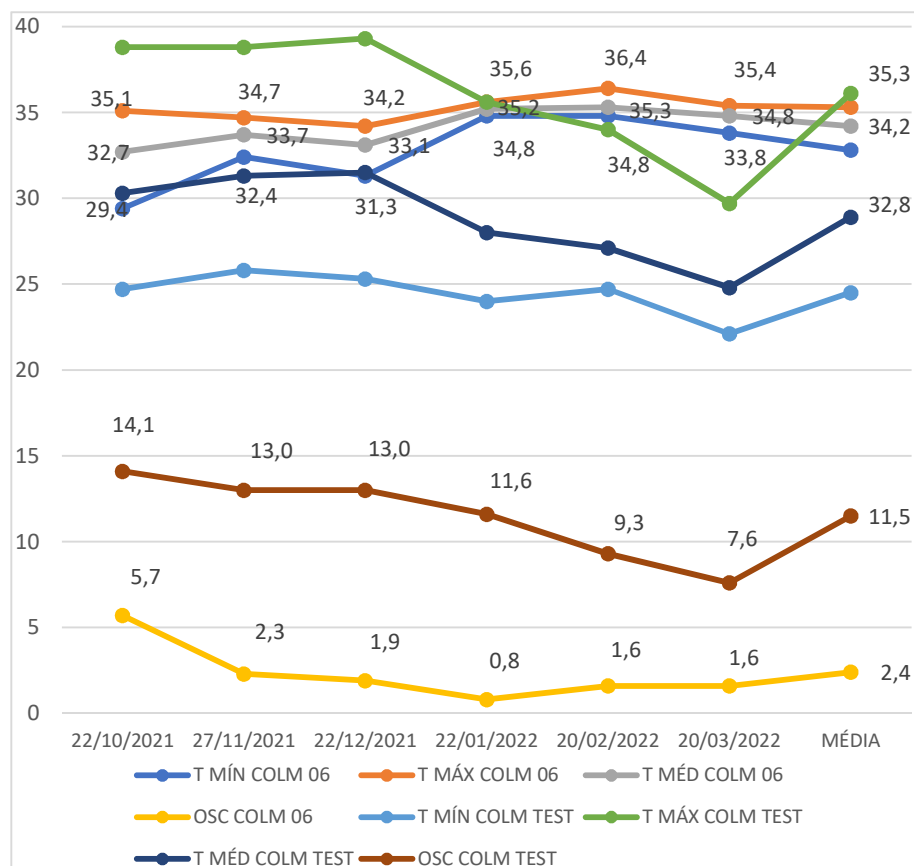
Gráfico 48 - Temperaturas registradas na colmeia 6 (povoada) e na colmeia 11 (testemunha) de out/2021 a mar/2022
