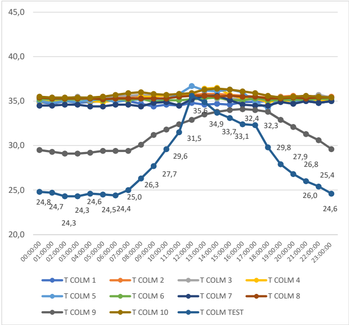
Gráfico 27 - Temperaturas e suas oscilações registradas nas colmeias povoadas e na colmeia testemunha, nas 24 (vinte e quatro) horas do dia 22 de janeiro de 2022 Fonte: Autor (2022)
