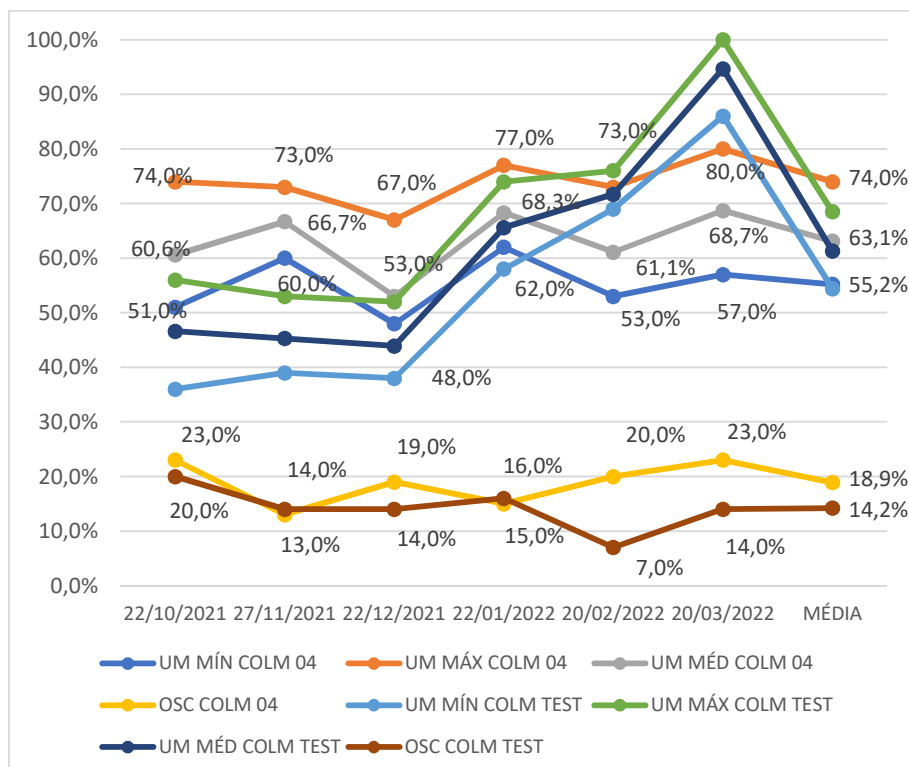
Gráfico 45 - Umidades registradas nas colmeias 4 (povoada) e na colmeia 11 (testemunha) de out/2021 a mar/2022 Fonte: Autor (2022)
