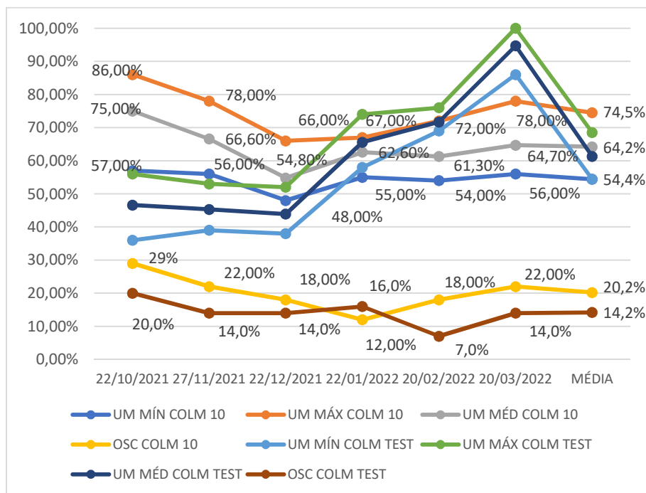
Gráfico 57 - Umidades registradas na colmeia 10 (povoada) e na colmeia 11 (testemunha), de out/2021 a mar/2022 Fonte: Autor (2022)
