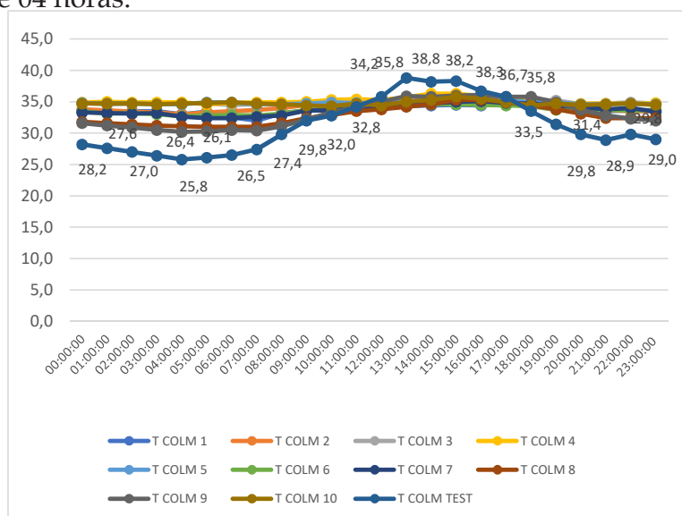
Gráfico 19 - Temperaturas e suas oscilações registradas nas colmeias povoadas e na colmeia testemunha, nas 24 (vinte e quatro) horas do dia 27 de novembro de 2021
