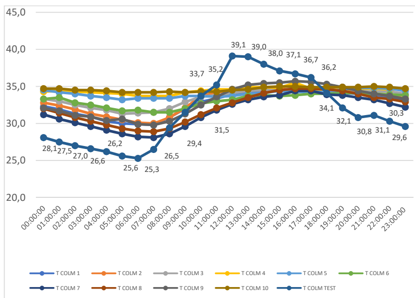
Gráfico 23 - Temperaturas e suas oscilações registradas nas colmeias povoadas e na colmeia testemunha, nas 24 (vinte e quatro) horas do dia 22 de dezembro de 2021
