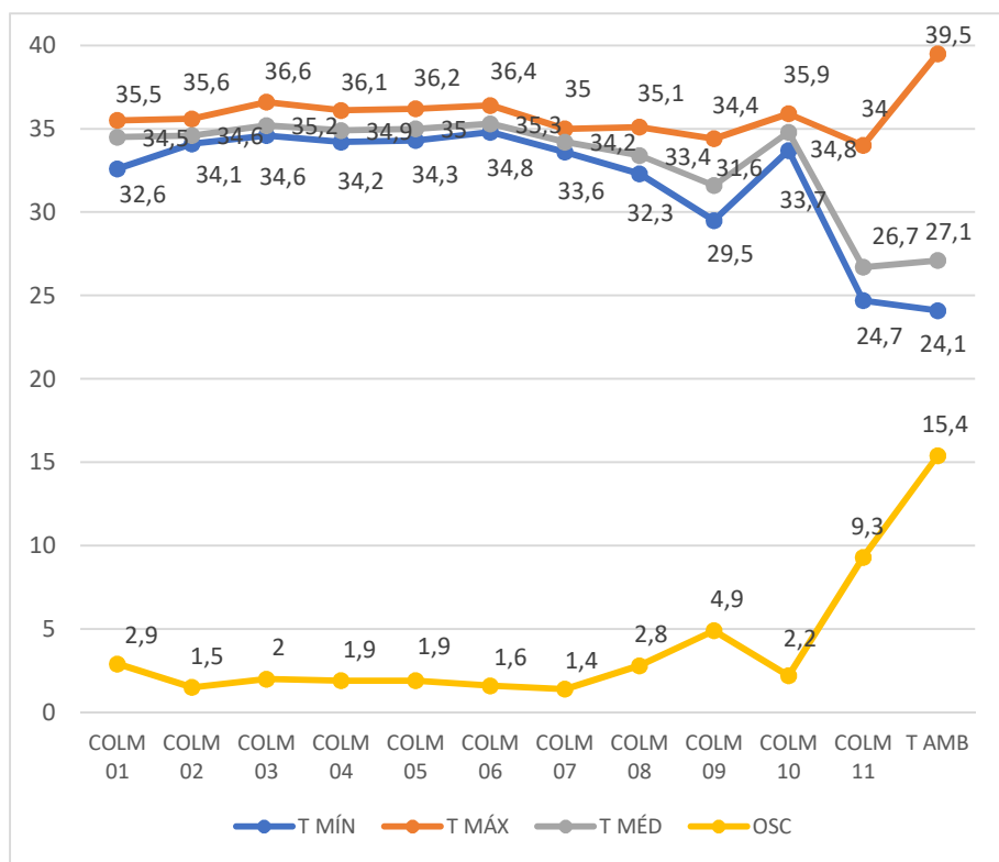
Gráfico 62 - Temperaturas mínima, máxima, média e as respectivas oscilações da temperatura na colmeia testemunha, no ambiente e nas dez colmeias povoadas, em 20/02/2022 Fonte: Autor (2022)
