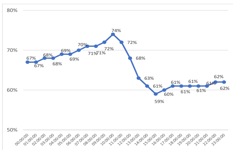
Gráfico 28 - Variação da Umidade na Colmeia 11 (Testemunha) em 22/01/2022 Fonte: Autor (2022)
