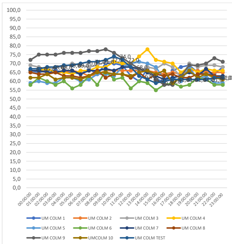
Gráfico 29 – Umidades e suas oscilações registradas nas colmeias povoadas e na colmeia testemunha, nas 24 (vinte e quatro) horas do dia 22 de janeiro de 2022 Fonte: Autor (2022)
