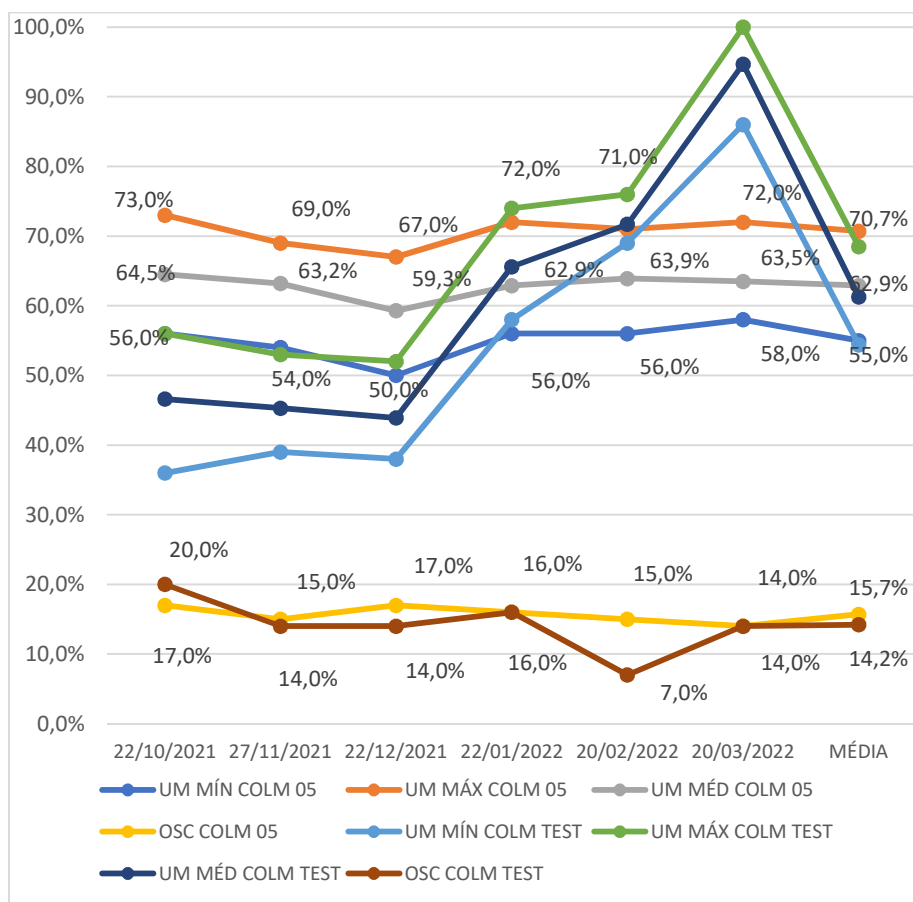
Gráfico 47 - Umidades registradas nas colmeias 5 (povoada) e na colmeia 11 (testemunha), de out/2021 a mar/2022
