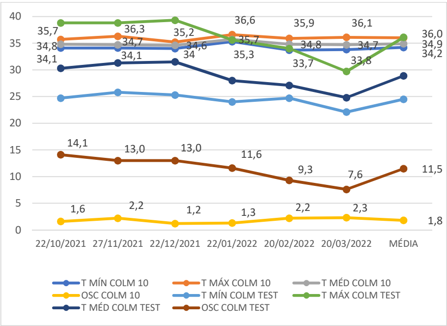
Gráfico 56 - Temperaturas registradas na colmeia 10 (povoada) e na colmeia 11 (testemunha) de out/2021 a mar/2022 Fonte: Autor (2022)
