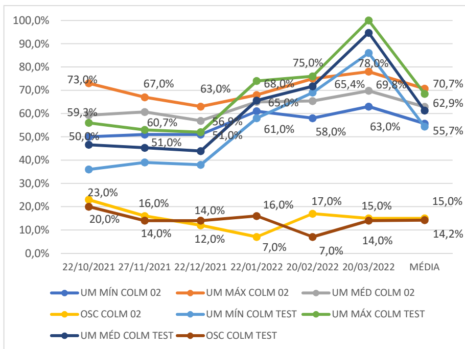
Gráfico 41 - Umidades registradas nas colmeias 2 (povoada) e na colmeia 11 (testemunha) de out/2021 a mar/2022 Fonte: Autor (2022)
