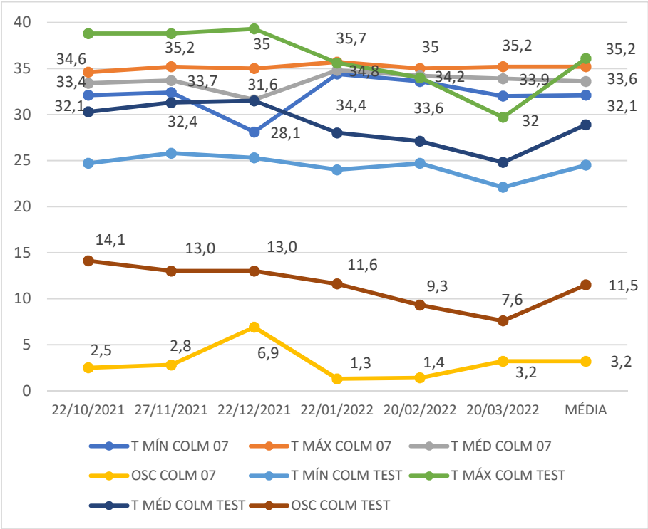
Gráfico 50 - Temperaturas registradas na colmeia 7 (povoada) e na colmeia 11 (testemunha) de out/2021 a mar/2022 Fonte: Autor (2022)
