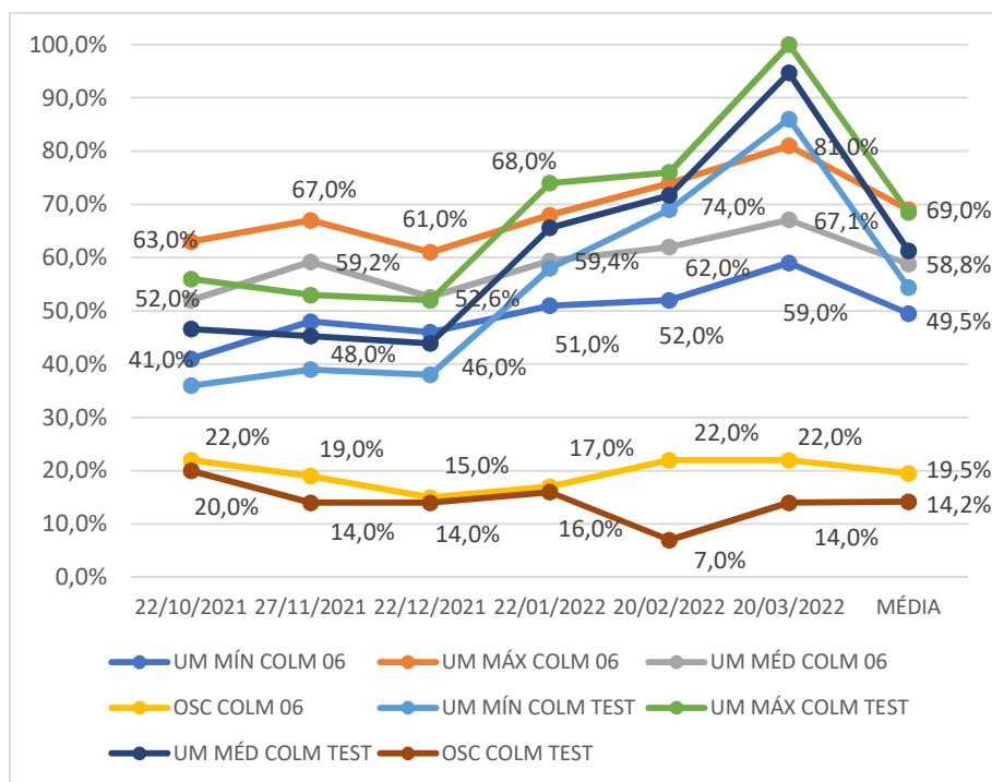
Gráfico 49 - Umidades registradas na colmeia 6 (povoada) e na colmeia 11 (testemunha), de out/2021 a mar/2022
