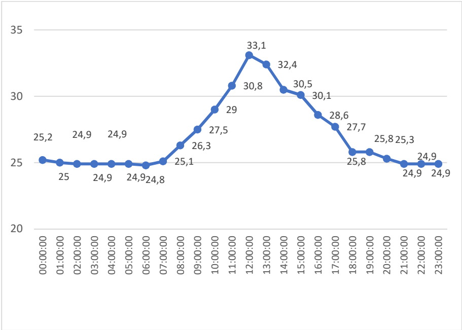
Gráfico 30 - Variação da temperatura na colmeia 11 (testemunha) em 20/02/2022 Fonte: Autor (2022)
