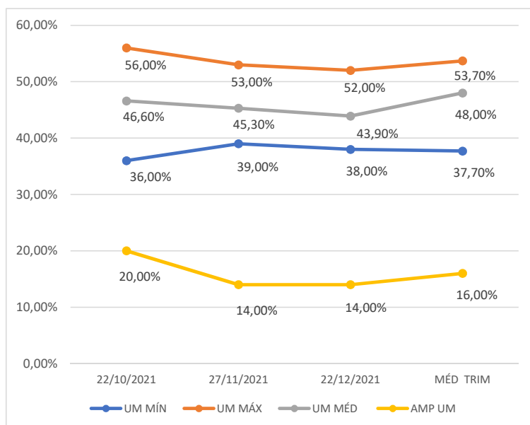
Gráfico 8 - Médias das umidades mínima, máxima, média e oscilação da umidade, registradas nos meses de outubro a dezembro de 2021 e a média desse trimestre
