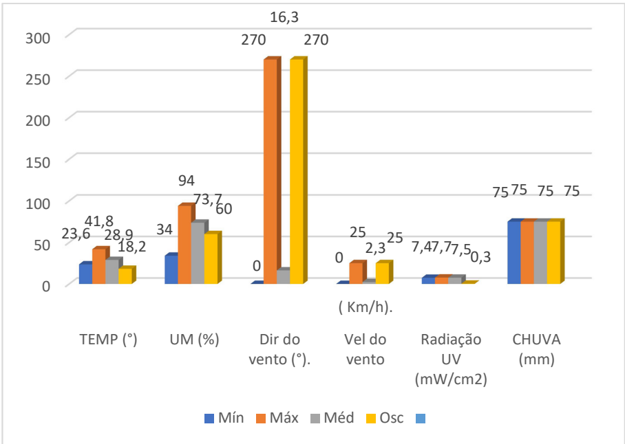
Gráfico 4 - Temperaturas, umidades, direção do vento, velocidade do vento, radiação UV e dados pluviométricos registrados nas estações 01 e 02 em 20/04/2022
