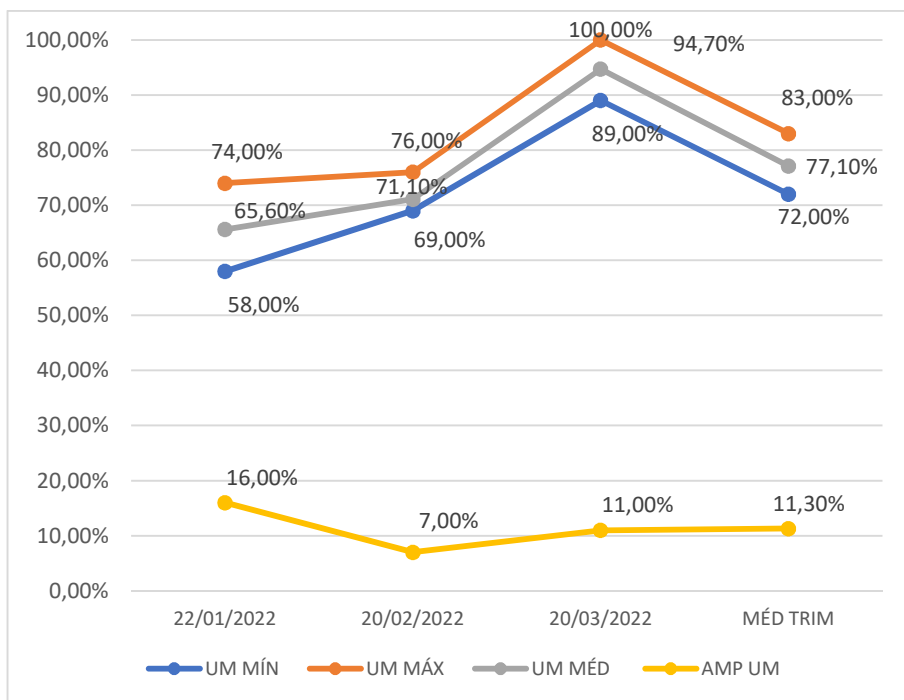
Gráfico 9 - Médias das umidades mínima, máxima, média e oscilação da umidade, registradas nos meses de janeiro a março de 2022 e a média desse trimestre
