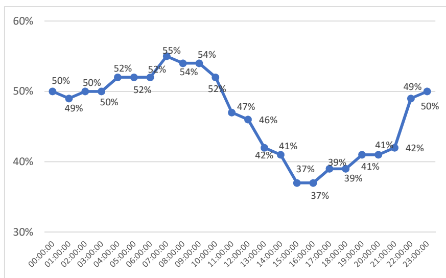
Gráfico 16 - Variação da umidade na colmeia 11(testemunha) em 22/10/2021 Fonte: Autor (2022)
