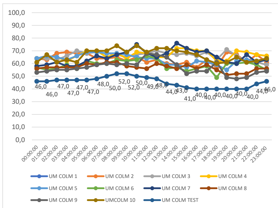
Gráfico 21 - Umidades e suas oscilações registradas nas colmeias povoadas e na colmeia testemunha, nas 24 (vinte e quatro) horas do dia 27 de novembro de 2021 Fonte: Autor (2022)
