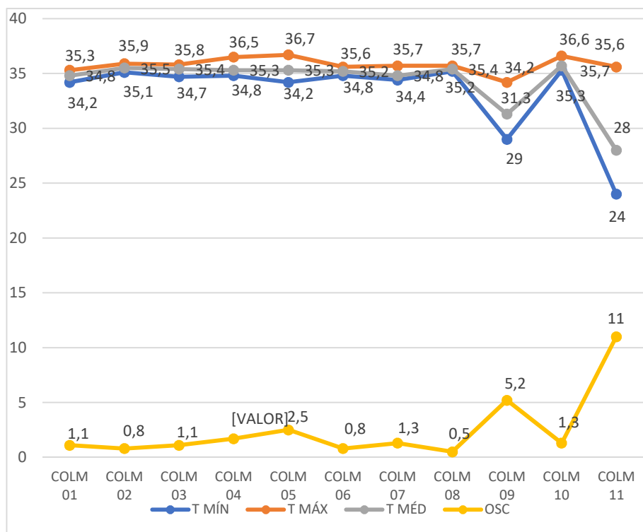
Gráfico 61 - Temperaturas mínima, máxima, média e as respectivas oscilações da temperatura na colmeia testemunha e nas dez colmeias povoadas, em 22/01/2022 Fonte: Autor (2022)
