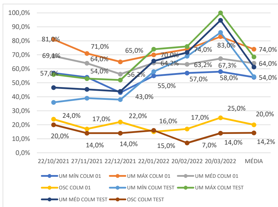
Gráfico 39 - Umidades registradas nas colmeias 01 e na colmeia 11 (testemunha) de out/2021 a mar/2022 Fonte: Autor (2022)
