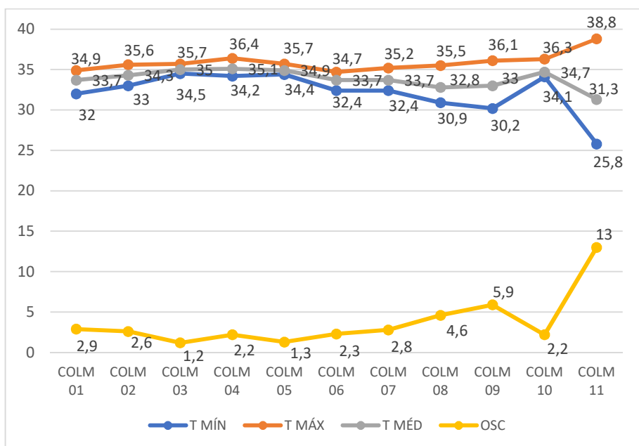
Gráfico 59 - Temperaturas mínima, máxima, média e as respectivas oscilações da temperatura na colmeia testemunha e nas dez colmeias povoadas, em 27/11/2021
