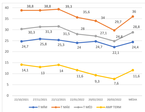
Gráfico 6 - Temperaturas mínima, máxima e média registradas na colmeia 11 (testemunha) de out/21 a mar/22 (três meses secos e três meses chuvosos) e a média do semestre Fonte: Autor (2022)
