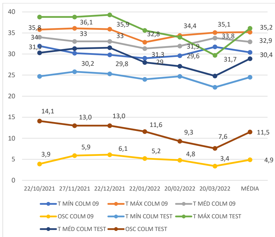
Gráfico 54 - Temperaturas registradas na colmeia 9 (povoada) e na colmeia 11 (testemunha) de out/2021 a mar/2022
