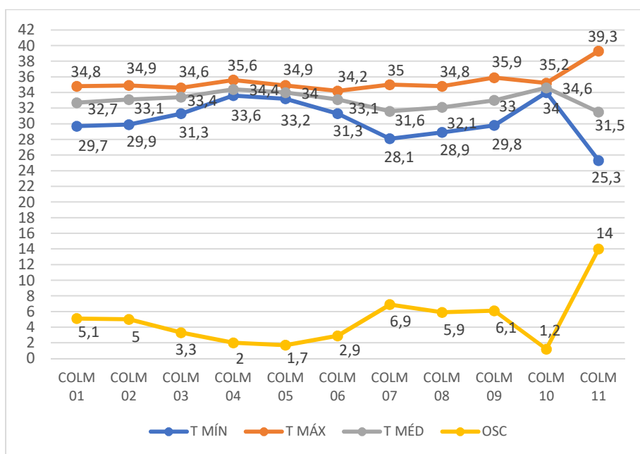
Gráfico 60 - temperaturas mínima, máxima, média e as respectivas oscilações da temperatura na colmeia testemunha e nas dez colmeias povoadas, em 22/12/2021
