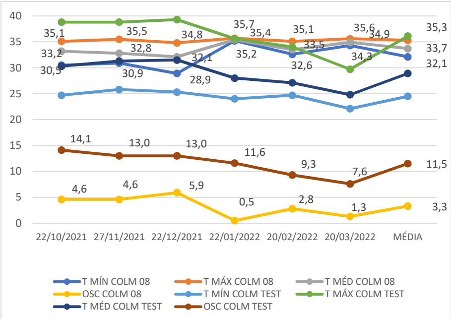
Gráfico 52 - Temperaturas registradas na colmeia 8 (povoada) e na colmeia 11 (testemunha) de out/2021 a mar/2022 Fonte: Autor (2022)
