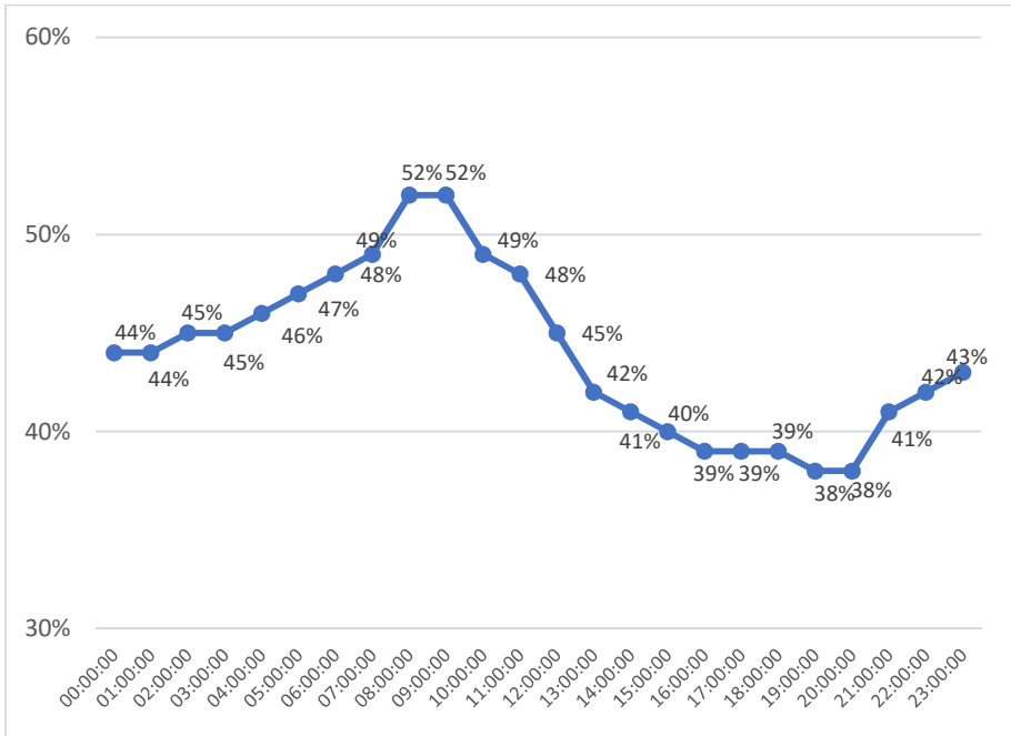
Gráfico 24 - Variação da umidade na colmeia 11 (testemunha) em 22/12/2021
