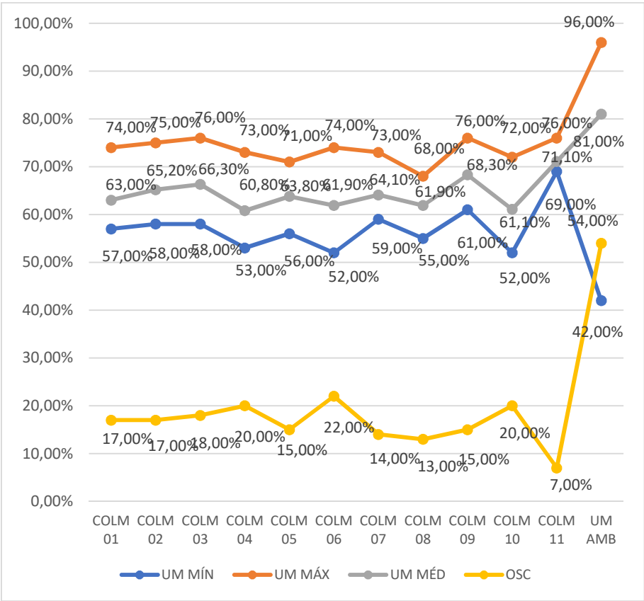
Gráfico 68 - Umidades mínima, máxima, média e as respectivas oscilações da umidade na colmeia testemunha, no ambiente e nas dez colmeias povoadas, em 20/02/2022 Fonte: Autor (2022)
