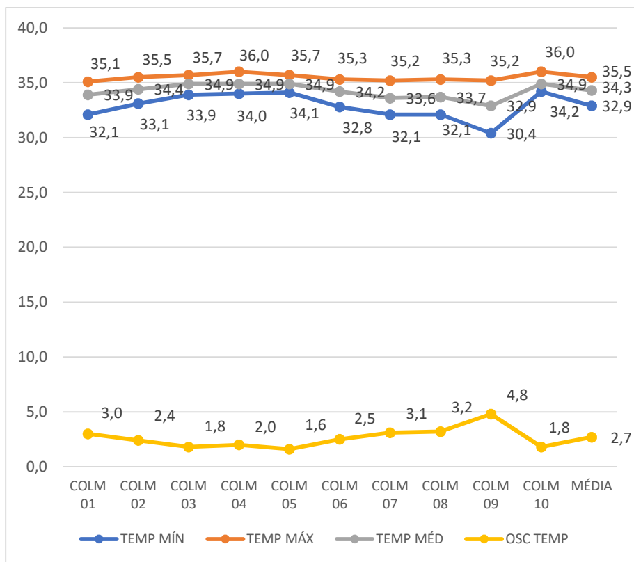
Gráfico 70 - Médias de temperatura mínima, máxima, média e a oscilação de temperatura, com dados dos seis meses pesquisados, das 10 colmeias para determinação da zona de conforto térmico no ninho da Apis mellifera L. Fonte: Autor (2022)
