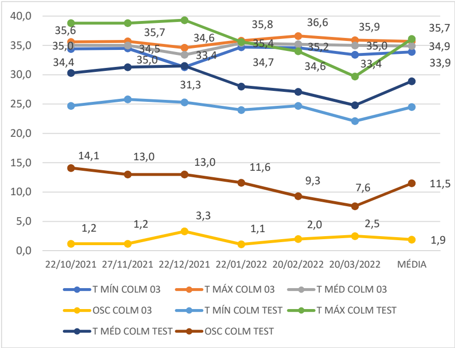
Gráfico 42 - Temperaturas registradas nas colmeias 3 (povoada) e na colmeia 11 (testemunha) de out/2021 a mar/2022 Fonte: Autor (2022)
