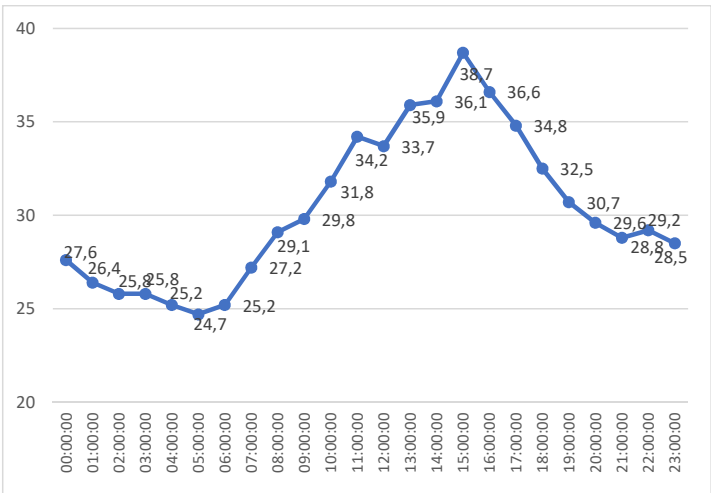
Gráfico 14 -Variação da temperatura na colmeia 11 (testemunha) em 22/10/2021 Fonte: Autor (2022)
