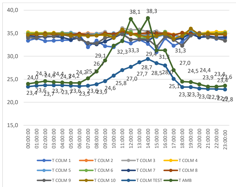
Gráfico 35 - Temperaturas e suas oscilações registradas nas colmeias povoadas, na colmeia testemunha e no ambiente, nas 24 (vinte e quatro) horas do dia 20 de março de 2022
