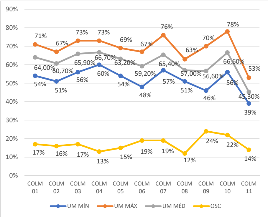
Gráfico 65 - Umidades mínima, máxima, média e as respectivas oscilações da umidade na colmeia testemunha, e nas dez colmeias povoadas, em 27/11/2022 Fonte: Autor (2022)
