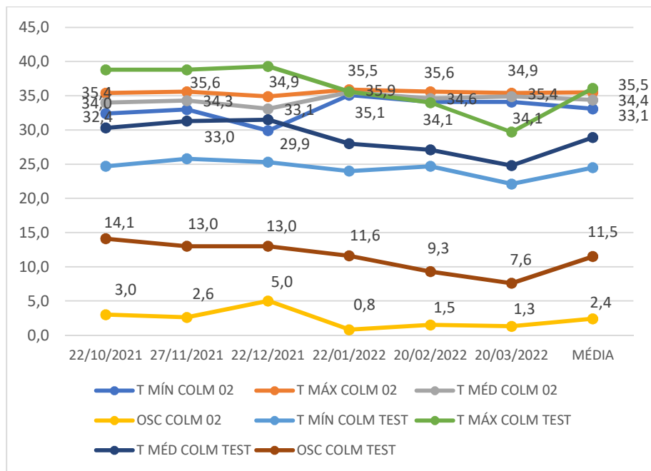
Gráfico 40 - Temperaturas registradas na colmeia 2 e na colmeia 11 (testemunha) de out/2021 a mar/2022 Fonte: Autor (2022)
