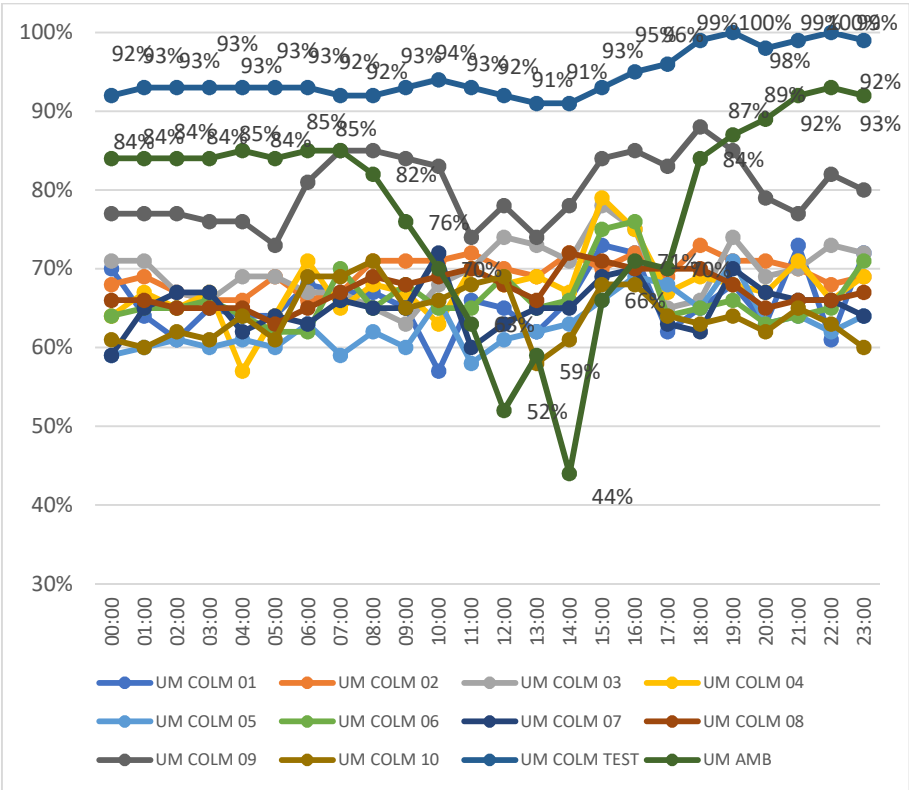
Gráfico 37 - Umidades e suas oscilações registradas nas colmeias povoadas, na colmeia testemunha e no ambiente, nas 24 (vinte e quatro) horas do dia 20 de março de 2022 Fonte: Autor (2022)
