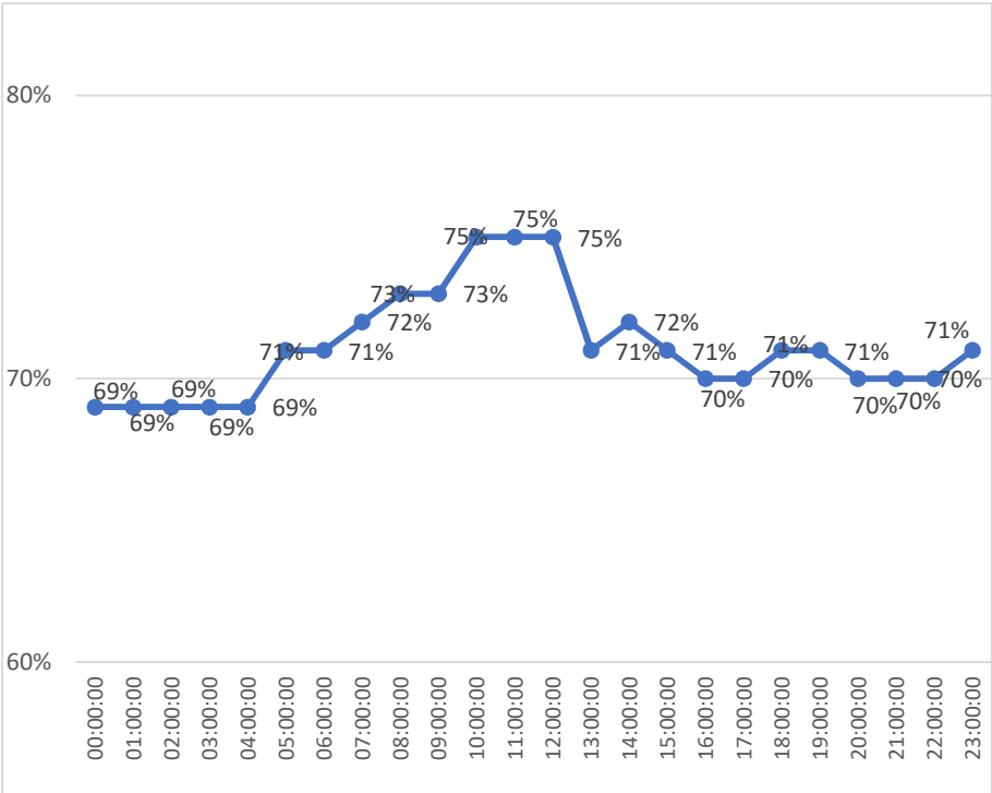
Gráfico 32 - Variação da umidade na colmeia 11 (testemunha) em 20/02/2022 Fonte: Autor (2022)
