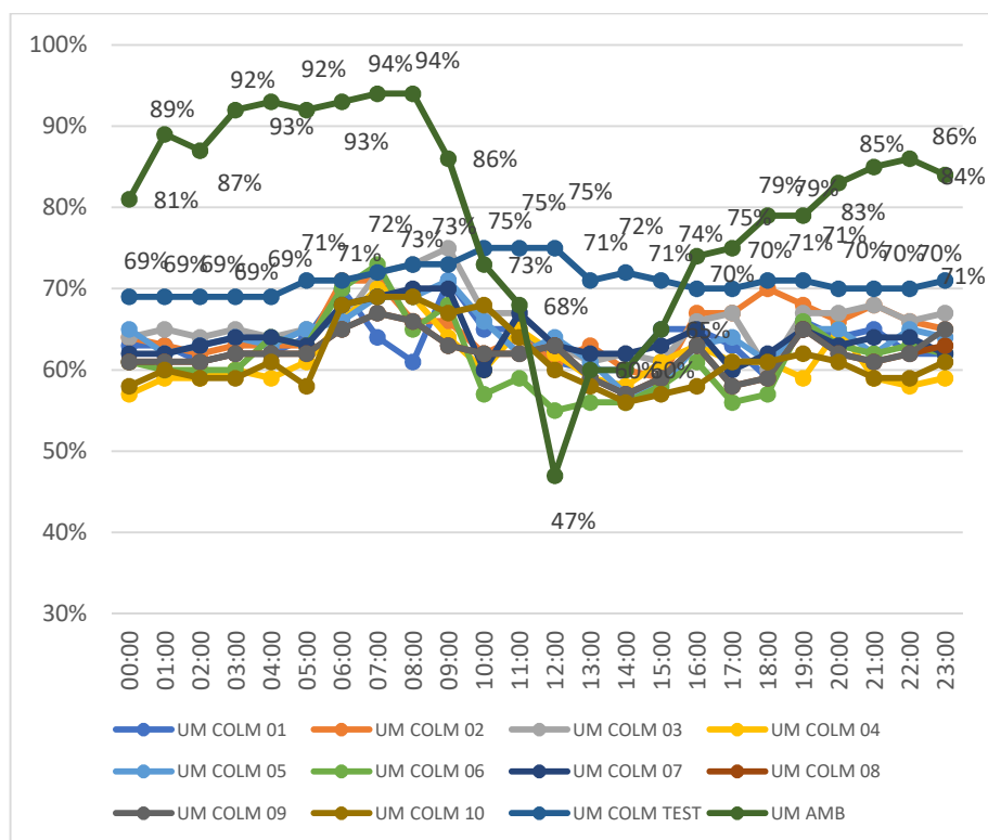
Gráfico 33 - Umidades e suas oscilações registradas nas colmeias povoadas, na colmeia testemunha e no ambiente, nas 24 (vinte e quatro) horas do dia 20 de fevereiro de 2022
