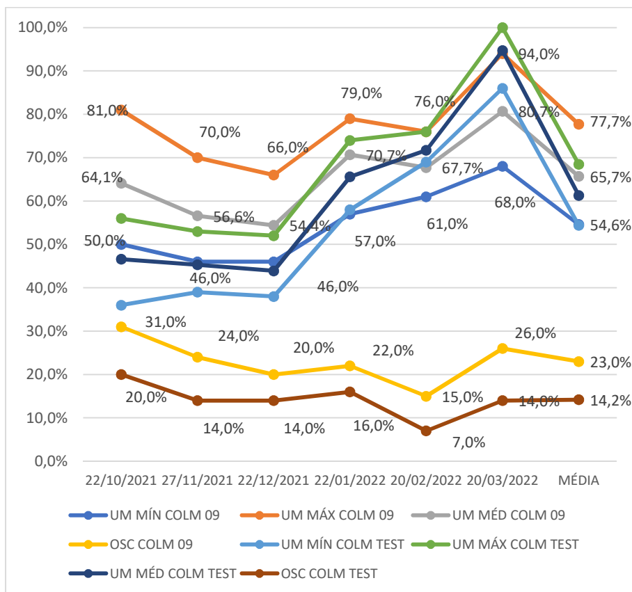
Gráfico 55 - Umidades registradas na colmeia 9 (povoada) e na colmeia 11 (testemunha), de out/2021 a mar/2022 Fonte: Autor (2022)
