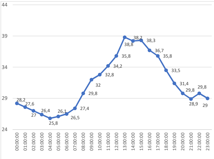
Gráfico 18 - Variação da temperatura na colmeia 11 (testemunha) em 27/11/2021 Fonte: Autor (2022)
