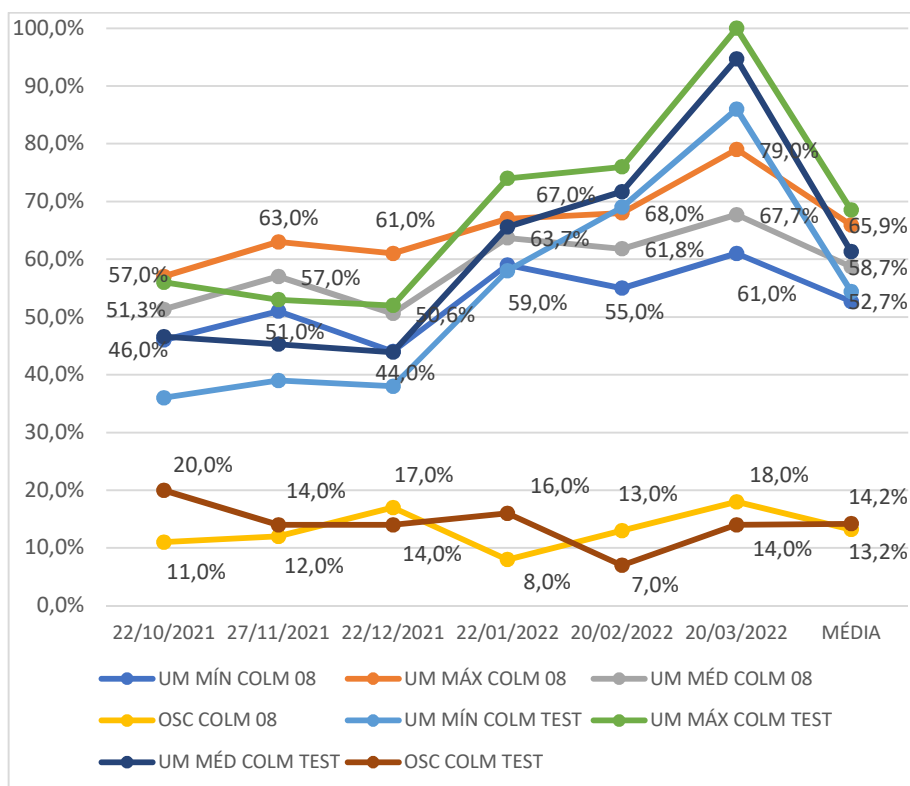
Gráfico 53 - Umidades registradas na colmeia 8 (povoada) e na colmeia 11 (testemunha), de out/2021 a mar/2022
