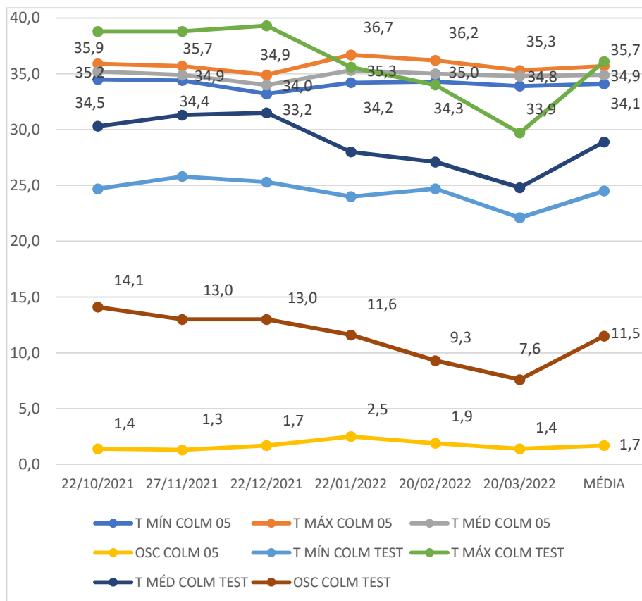
Gráfico 46 - Temperaturas registradas na colmeia 5 (povoada) e na colmeia 11 (testemunha) de out/2021 a mar/2022
