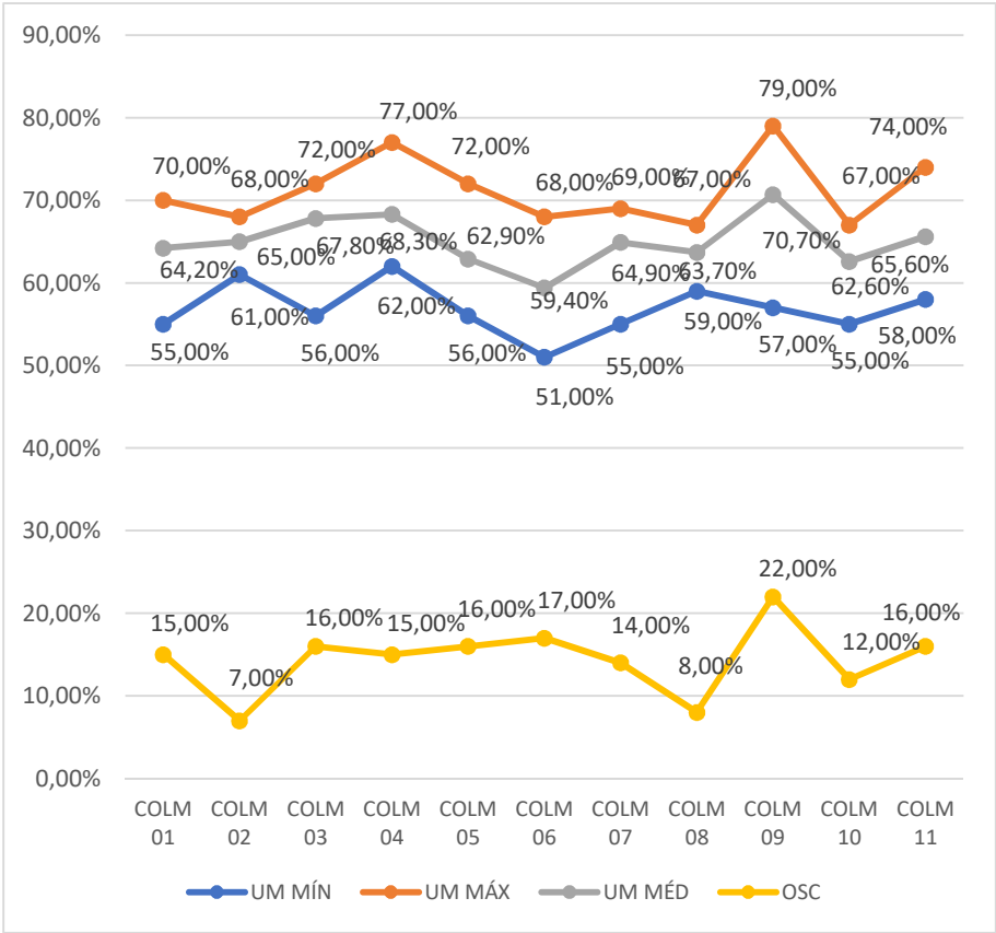
Gráfico 67 - Umidades mínima, máxima, média e as respectivas oscilações da umidade na colmeia testemunha, e nas dez colmeias povoadas, em 22/01/2022 Fonte: Autor (2022)
