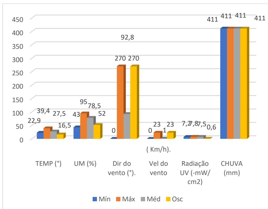
Gráfico 3 - Temperaturas, umidades, direção do vento, velocidade do vento, radiação UV e dados pluviométricos registrados nas estações 01 e 02 em 20/03/2022
